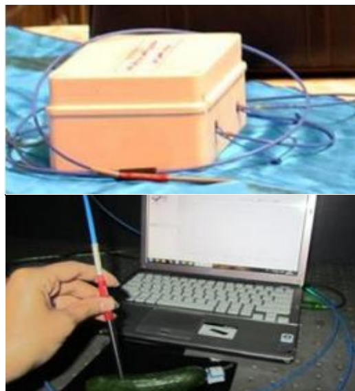
شکل ۵- سامانه اپتیکی تشخیص و تعیین سریع و غیرمخرب باقیمانده سموم در محصول [۱]
